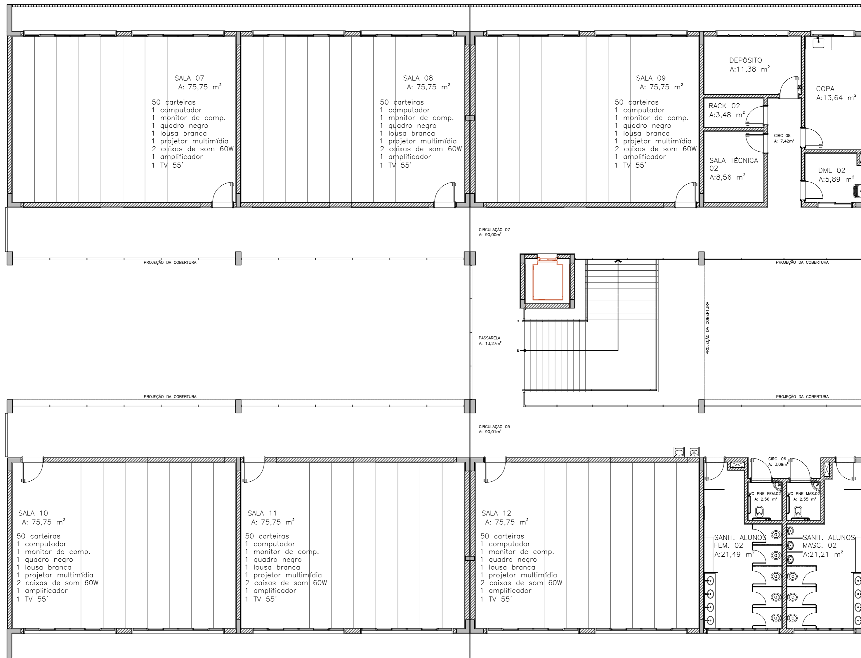
PAVILHÃO DE AULA 9 – Segundo Pavimento
