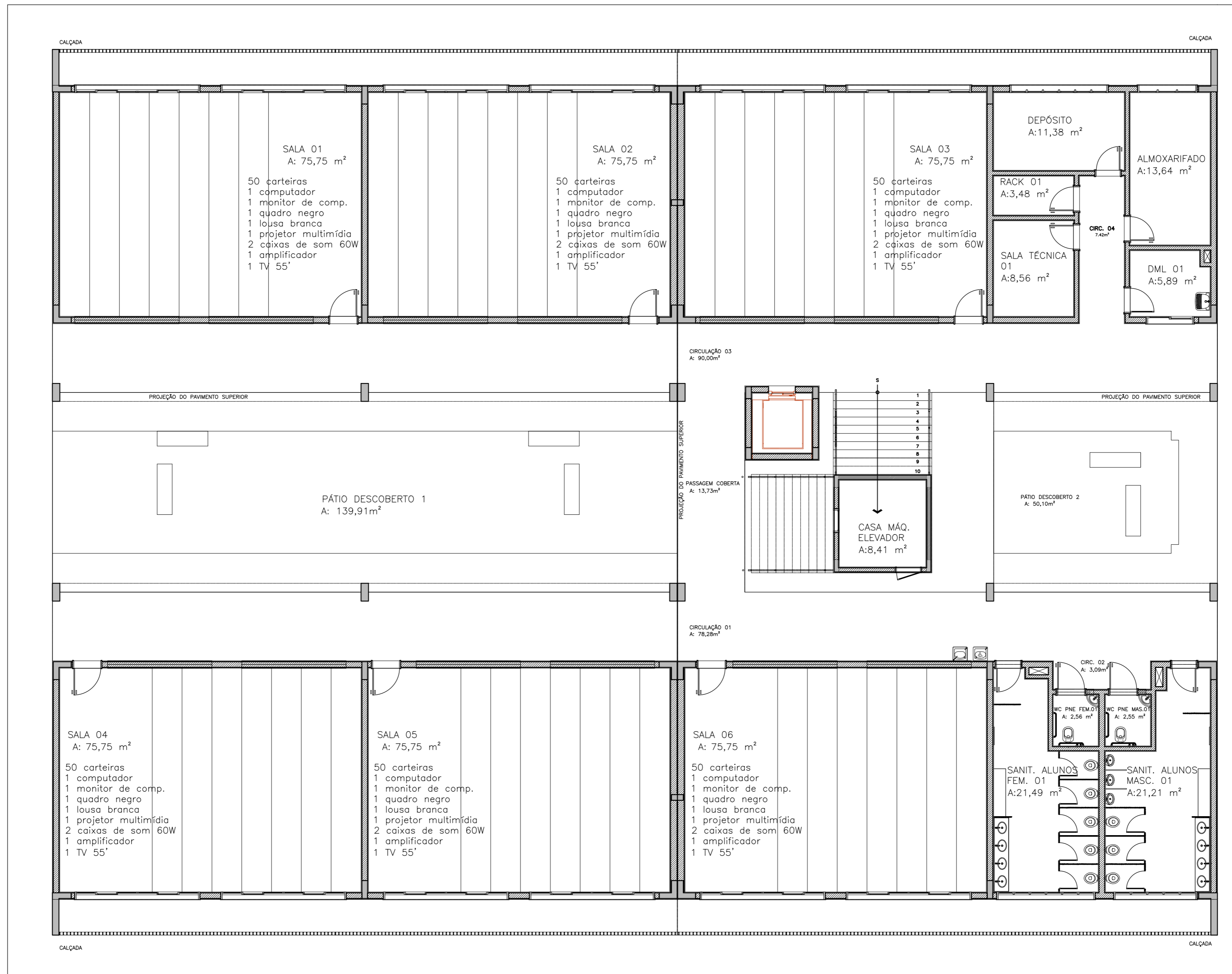
PAVILHÃO DE AULA 9 – Pavimento Térreo
