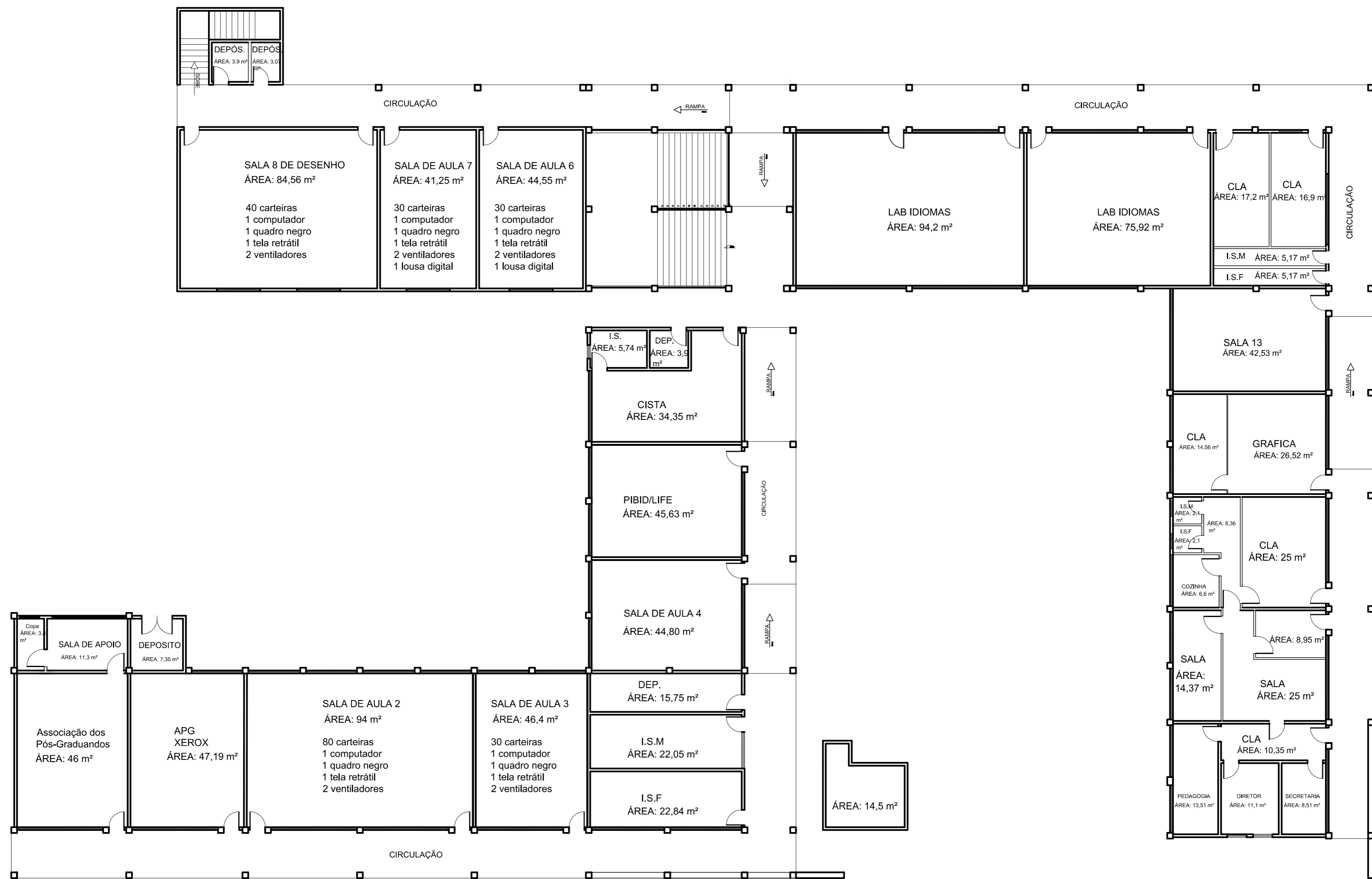
PAVILHÃO DE AULA 6 - TÉRREO ÁREA: 1653,21 m 2
